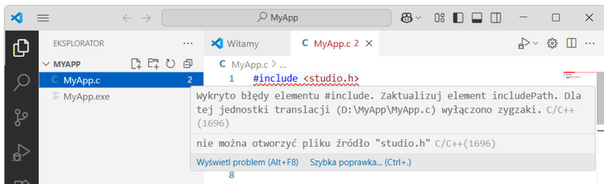
Rys. 31. Informacje o błędach po najechaniu kursorem myszki na podkreślenie
