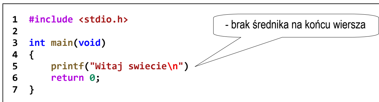
Rys. 31. Informacje o błędach po najechaniu kursorem myszki na podkreślenie
