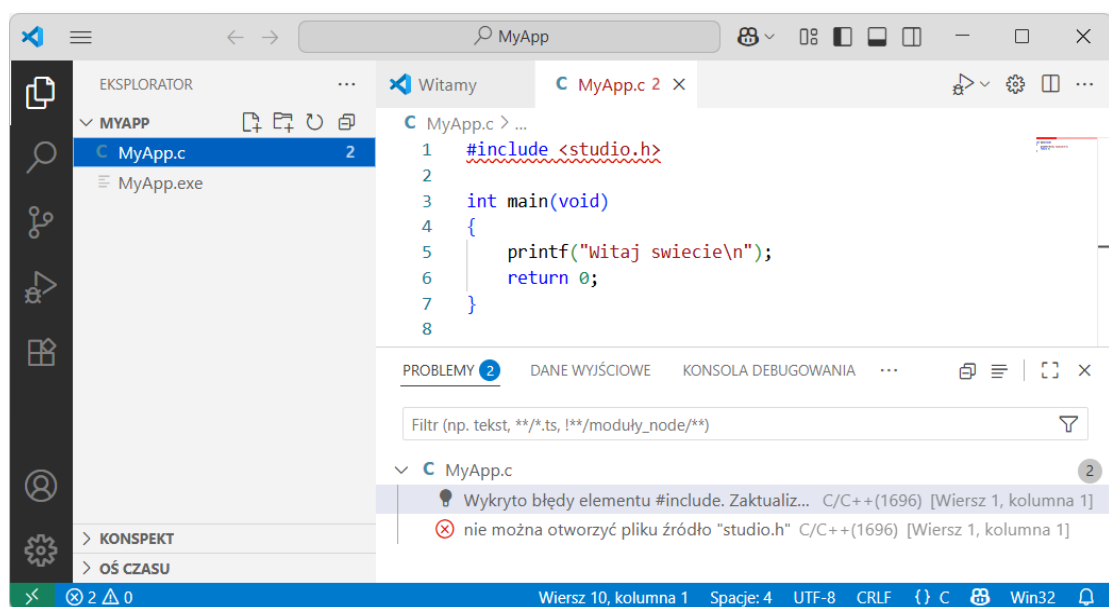
Rys. 30. Informacje o błędach w oknie PROBLEMY
