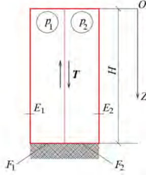
Rysunek 8.1: Układ statyczny złożony z dwóch pasm (opr. E. Koźniewski na podstawie [52])
