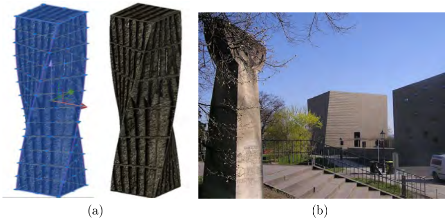
Rysunek 4.8: (a) skrócenie prostopadłościanu, krawędzie pionowe jako linie śrubowe (modele zrealizowane w AutoCAD-zie), opr. E. Koźniewski na podstawie [51]; (b) synagoga w Dreżnie (2001, architekci Rena Wandel-Hoefer oraz Wolfgang Lorch) – przykład zastosowania w architekturze przekształcenia skrócenie [18]
