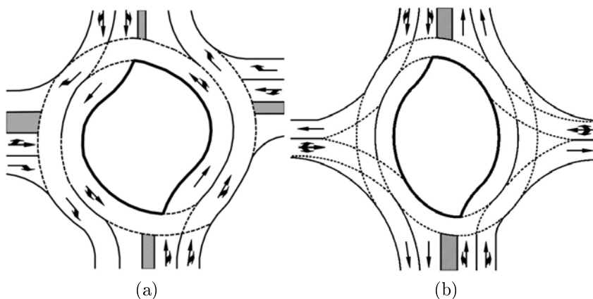
Rysunek 5.1: Szkic ronda turbinowego ukształtowanego za pomocą: (a) dwóch pół-okręgów, wyk. E. Koźniewski na podstawie [9]; (b) elipsy, wyk. E. Koźniewski na podstawie [9]
