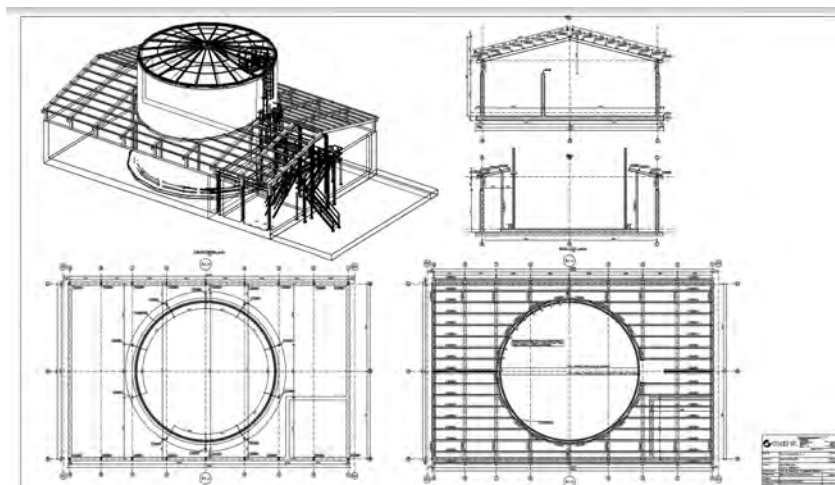
Rysunek 3.3: Projekt zadaszania zbiornika na paliwo (struktura powierzchni walcowej i stożkowej). Współpraca proj. B. Koźniewski
