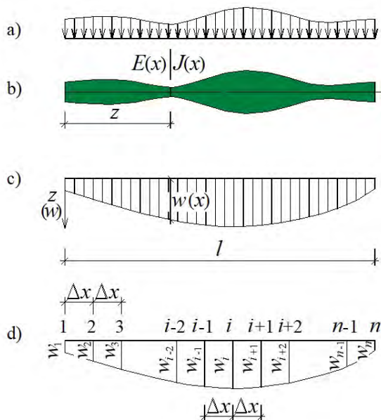
Rysunek 9.6: Metoda różnicowa. Model pręta zginanego, wyk. E. Koźniewski na podstawie [53]
