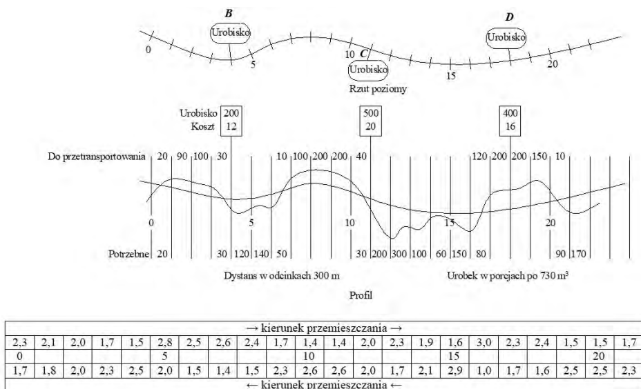
Rysunek 11.3: Prace ziemne przy budowie autostrady [56], opr. E. Koźniewski
