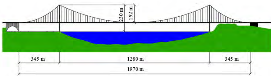
Rysunek 6.4: Podstawowe wymiary mostu wiszącego Golden Gate Bridge łączącego San Francisco z Marin County w Kalifornii (USA), wyk. E. Koźniewski na podstawie [23]
