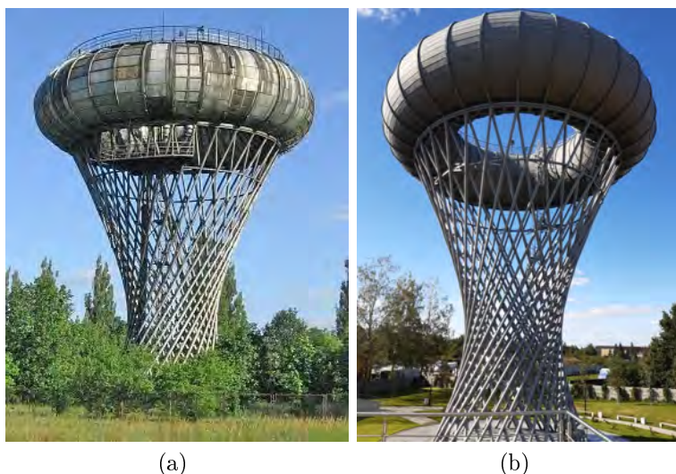
Rysunek 3.4: Budowle w kształcie hiperboloidy: (a) wieża ciśnień w Ciechanowie – struktura nośna w kształcie hiperboloidy jednopowłokowej i zbiornik w kształcie torusa – stan przed renowacją; (b) wieża ciśnień w Ciechanowie po renowacji jako główny element parku nauki, fot. B. Koźniewski
