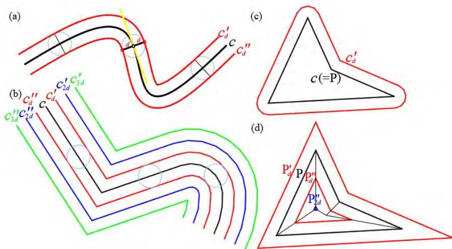
Rysunek 5.2: Offsety: (a) krzywej sklepanej; (b) polilinii; (c) półoffset wielokąta (otrzymany za pomocą programu AutoCAD ze stałą Offsetgaptype = 1); (d) dyskretne półoffsety wielokąta (otrzymany za pomocą programu AutoCAD ze stałą Offsetgaptype = 0), opr. E. Koźniewski
