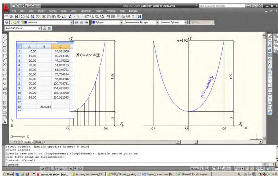
Rysunek 6.3: Generowanie profilu krzywej łańcuchowej w programie AutoCAD: punkty wyznaczone dla krzywej łańcuchowej (6.8) dla a = 38,9216 , dla wartości 10, 20, ..., 80, 90, 96 (pierwsza kolumna liczb), obliczając w Excelu wartości funkcji (6.8) (druga kolumna) i odmierzając je na prostych pionowych wystawionych w punktach o odciętych 10, 20, ..., opr. E. Koźniewski
