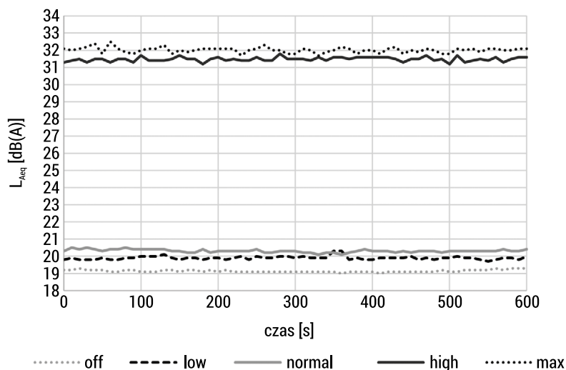
RYS. 4. Zmienność równoważnego poziomu dźwięku L_{Aeq} dla różnych nastaw wentylatora (OFF–MAX) – pomiar 2
