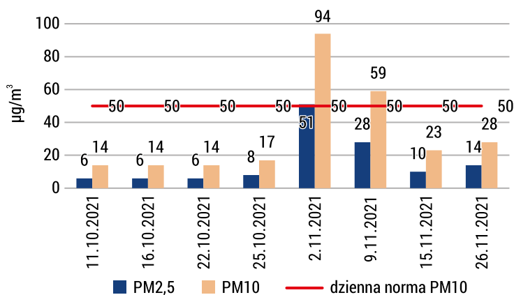
RYS. 7. Wyniki pomiarów stężenia pyłów \text{PM}_{2,5} i \text{PM}_{10} w powietrzu w punkcie pomiarowym nr 5
