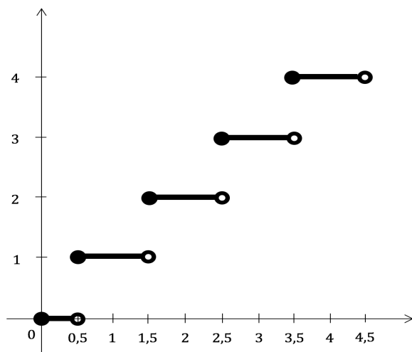
Rysunek 3.1: Wykres funkcji (r)_0
