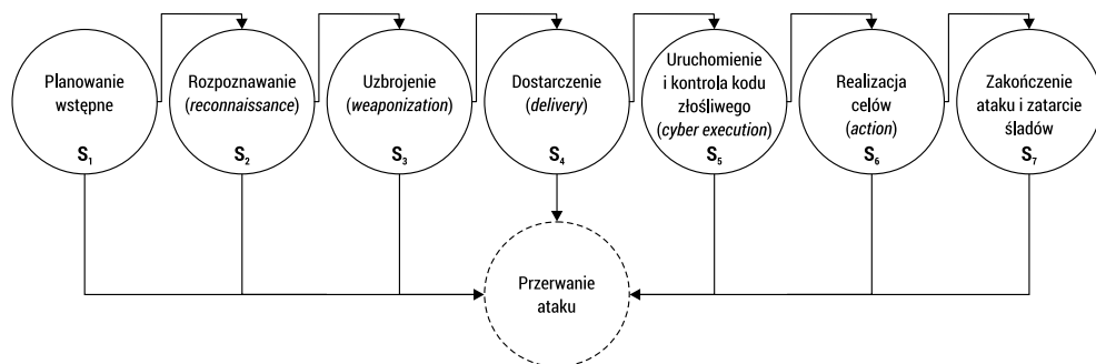
RYŚ. 1. Graf przejść pomiędzy fazami ogólnego cyklu życia ataku cybernetycznego
