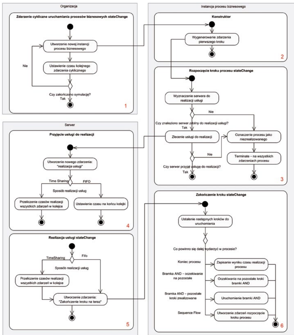
RYS. 2. Algorytm działania symulatora
