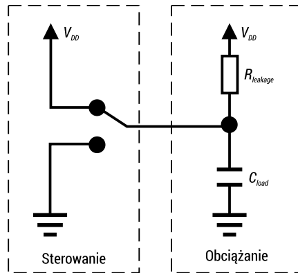
RYS. 1. Uproszczony schemat inwertera CMOS (na podstawie [12])
