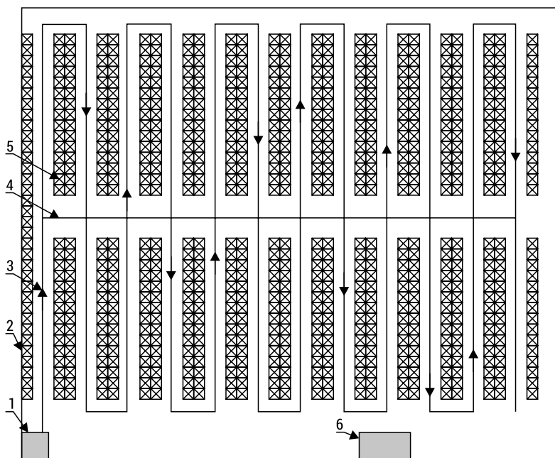
RYS. 9. Schemat magazynu: 1 – strefa rozpoczęcia kompletacji, 2 – paleta z materiałem, 3 – droga kompletacji, 4 – droga komunikacyjna, 5 – regał przesuwany, 6 – miejsce odkładania skompletowanych zamówień
