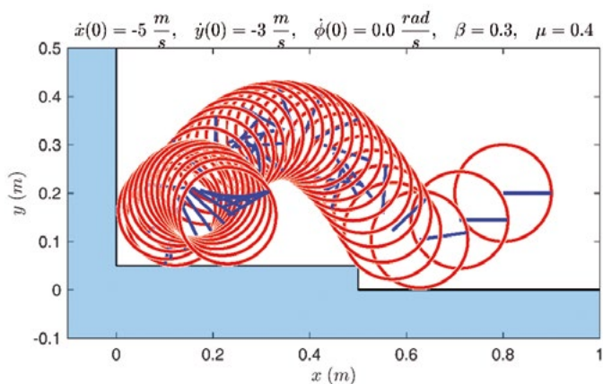
RYS. 11. Sekwencja położenia koła w trakcie symulacji (zderzenia sprężysto-plastyczne)
