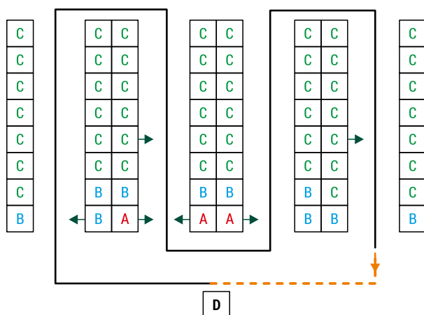
RYS. 1. Strategia Across-Aisle z metodą przejścia S-Shape
