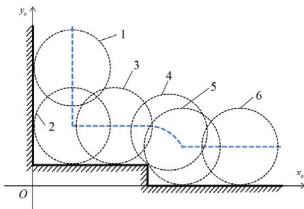
RYS. 3. Sześć szczególnych położeń, w których koło styka się z brzegiem ograniczenia
