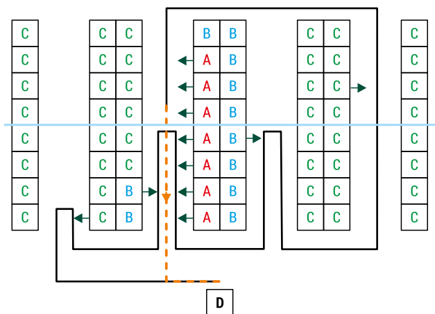
RYS. 4. Strategia Within-Aisle z metodą przejścia Midpoint
