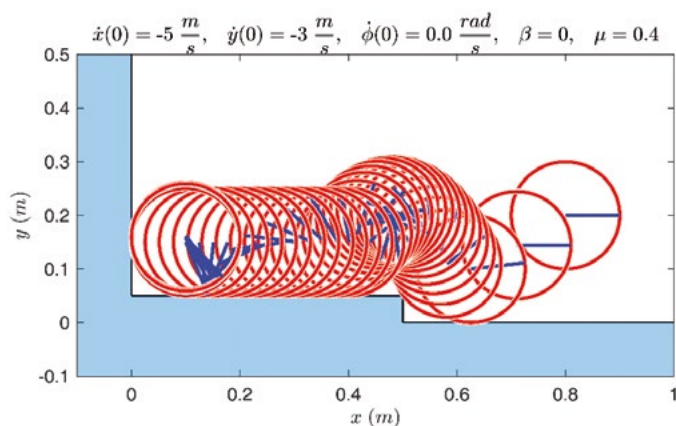
RYS. 10. Sekwencja położenia koła w trakcie symulacji (zderzenia plastyczne)
