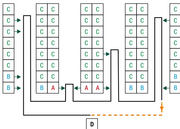
RYS. 3. Strategia Perimeter Storage z metodą przejścia Return
