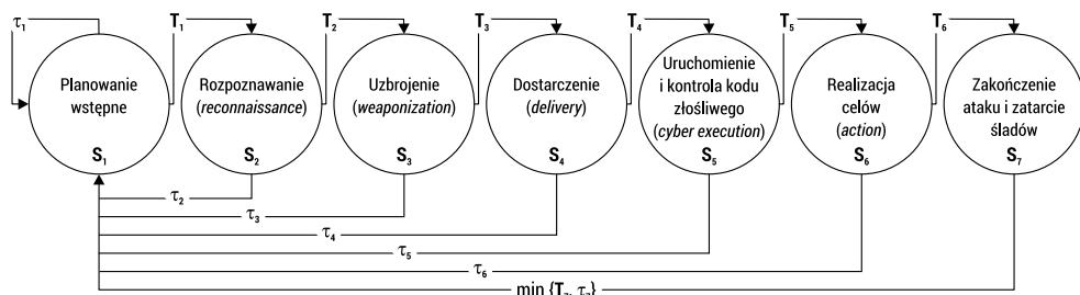
RYS. 2. Graf ogólnego cyklu życia ataku cybernetycznego z czasami przebywania w fazach
