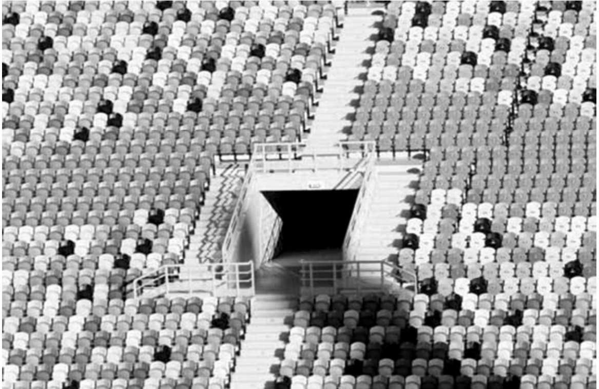
Fot. 4-6. Stadion im. Jose Alvalade , Lisboa. Fragment widowni – przykład aranżacji z osiowym układem schodów południkowych nad i poniżej womitorium. System pozwala na segregację pasm ruchu widzów w obrębie przestrzeni womitorium.
