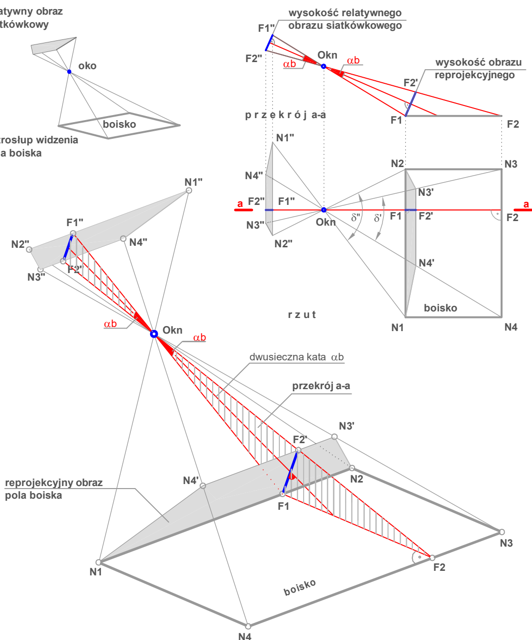
RYŚ. 2-6 "OSTROŚŁUP WIDZENIA" POLA BOISKA - PIONOWY KĄT WIDZENIA
