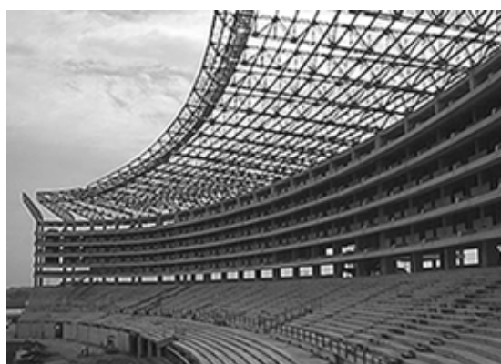
Fot. 1-32. (po lewej) Estadio Teodoro Fernandez (Monumental de la „U”) , Ate – Lima, Peru (2000). W Południowej Ameryce wykształca się obecnie ciekawy, niespotykany gdzie indziej, typ stadionu. Idea ta polega na zestawianiu dwóch rodzajów widowni – tradycyjnej dolnej i wielopiętrowej górnej, która składa się z indywidualnych łóż z zapleczem. Foto: www.universitariodedeportes.biz/index.php?historia .
