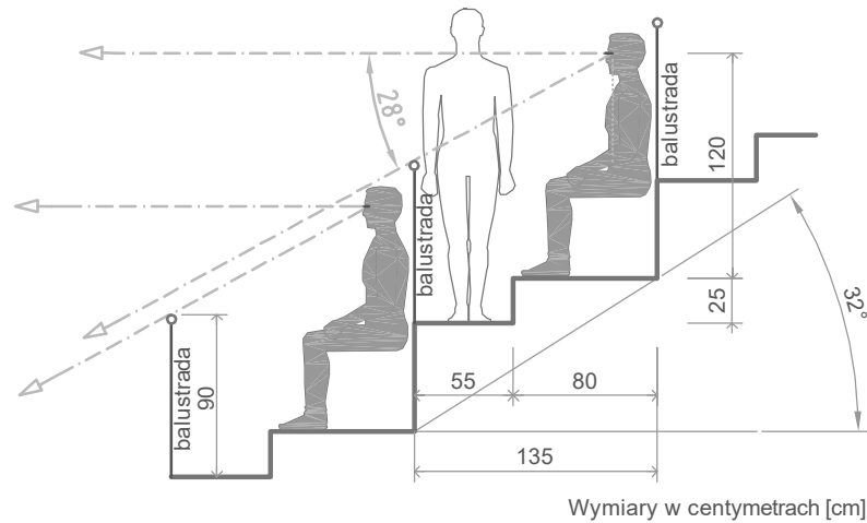
RYS. 5-1 TRYBUNA O PODWYŻSZONYM KOMFORTCIE UŻYTKOWYM - RZĄD Z BALUSTRADĄ I OBNIŻONYM PRZEJŚCIEM Z PRZODU
