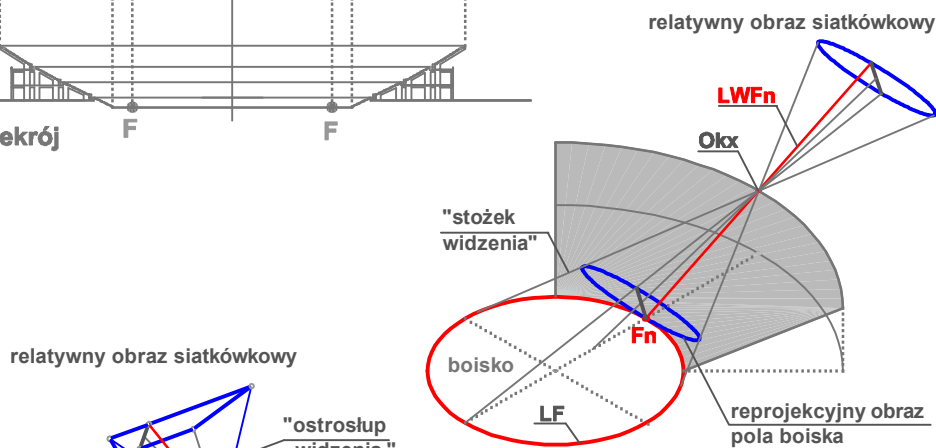
B.) BOISKO KOŁOWE - WIDOWNIA KOŁOWA
