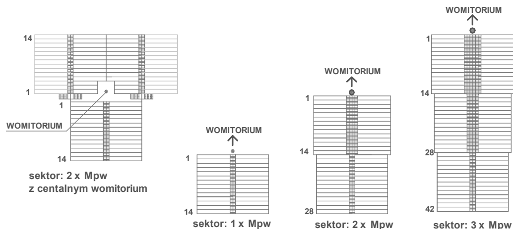
MODELOWE ZESTAWIENIA MODUŁÓW Mpw. Wstępne kształtowanie sektora widowni.
