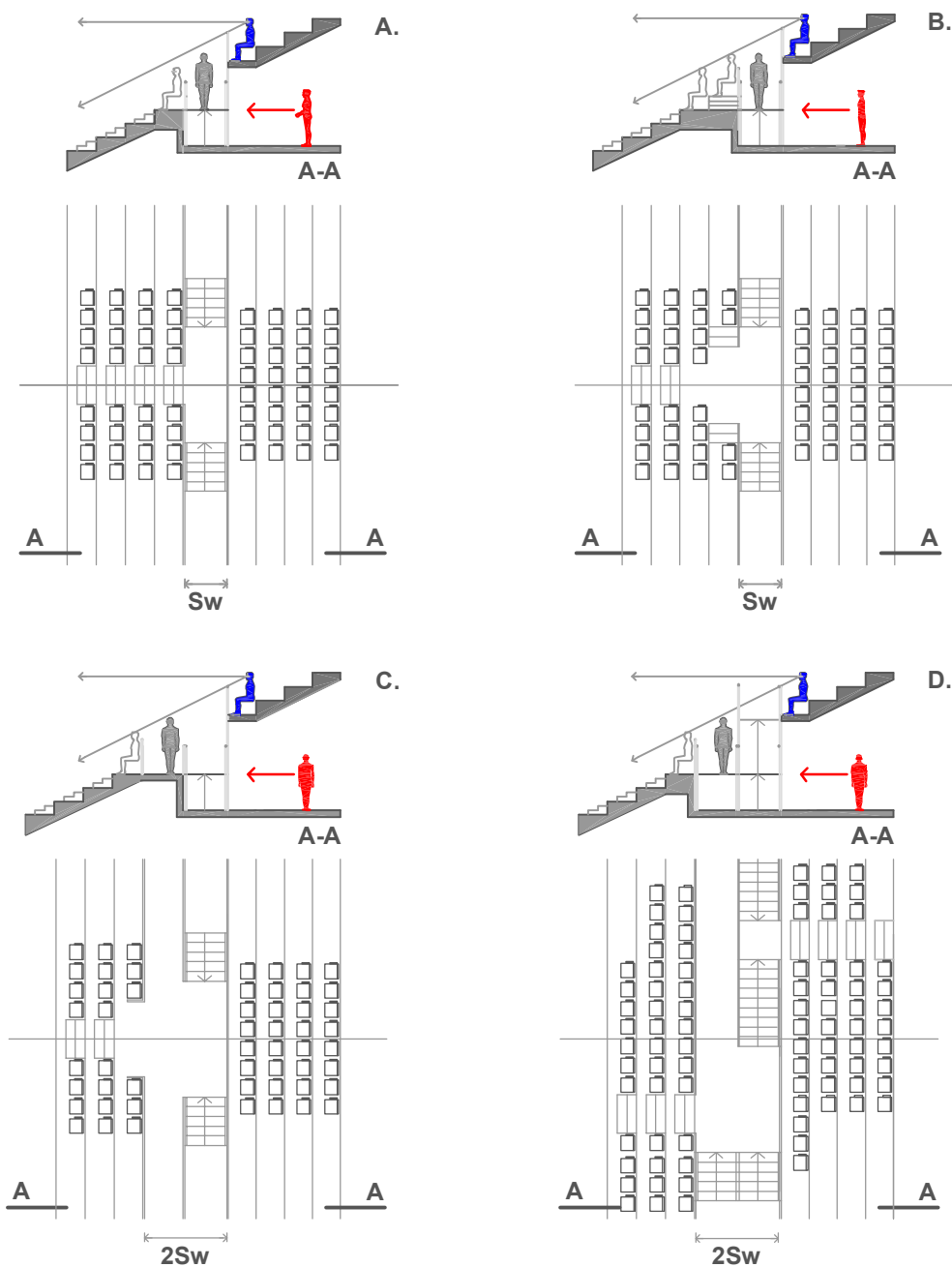
RYS. 5-6 WOMITORIA RÓWNOLEŻNIKOWE
