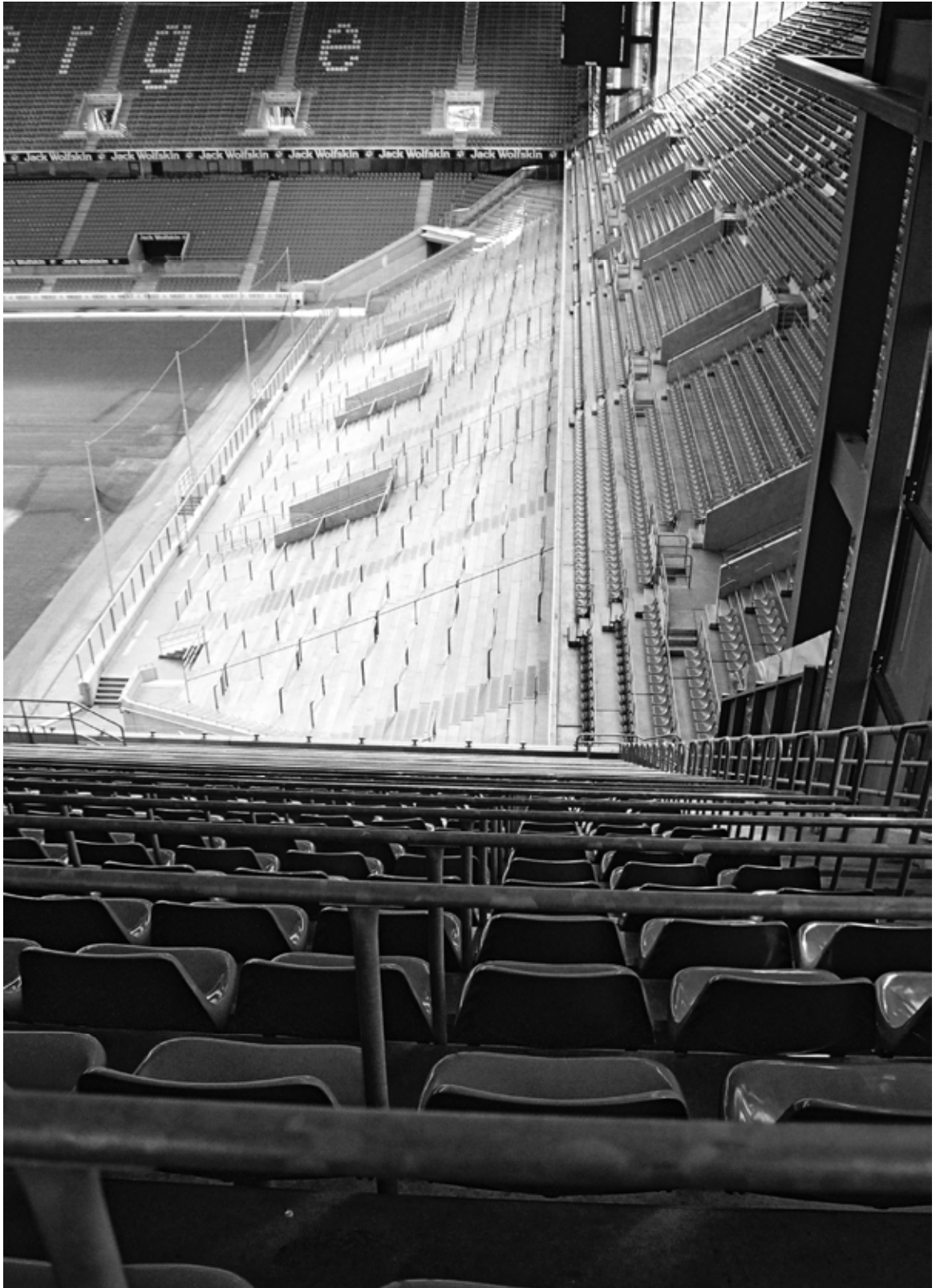
Fot. 2-7. RheinEnergy Stadion, Kolonia, (2004). Przykład widowni prostokątnej o profilu prostoliniowym. Nachylenie widowni górnej wynosi 35^\circ , co jest maksymalną normowo dopuszczalną wartością. Tak znaczna stromizna trybun wymagała zastosowania w każdym rzędzie balustrady czołowej. Niezwykłością prezentowanej widowni jest rozwiązanie trybun w rejonie narożnika boiska. Tak dalekie wysunięcie poza linię bramkową skrajnych miejsc powoduje, że mają one ekspozycję widokową nie na boisko lecz na prostopadłe trybuny. Nakierowanie centralnej linii widzenia na najbardziej skrajny narożnik obrazu pola boiska wymaga skręcenia tej osi o kąt dochodzący do wartości ok. 67^\circ . Foto: autor.
