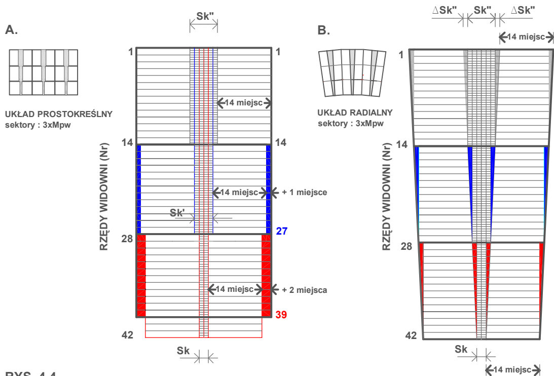
RYŚ. 4-4 PRZYKŁAD KSZTAŁTOWANIA POWTARZALNEGO SEKTORA WIDOWNI Z ZASTOSOWANIEM EWAKUACYJNEGO MODUŁU POJEMNOŚCI. A. Transformacja sektora 3xMpw dla widowni o układzie prostokreślnym. B. Transformacja sektora 3xMpw dla widowni o układzie radialnym
