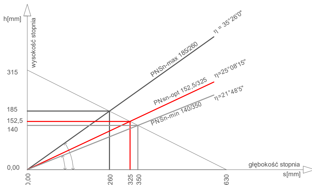
RYS. 3-3 GRANICZNE PARAMETRY STOPNI DLA SCHODÓW NORMALNYCH
