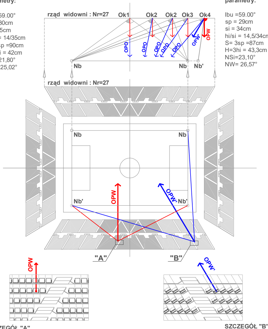
SZCZEGÓŁ "A"
