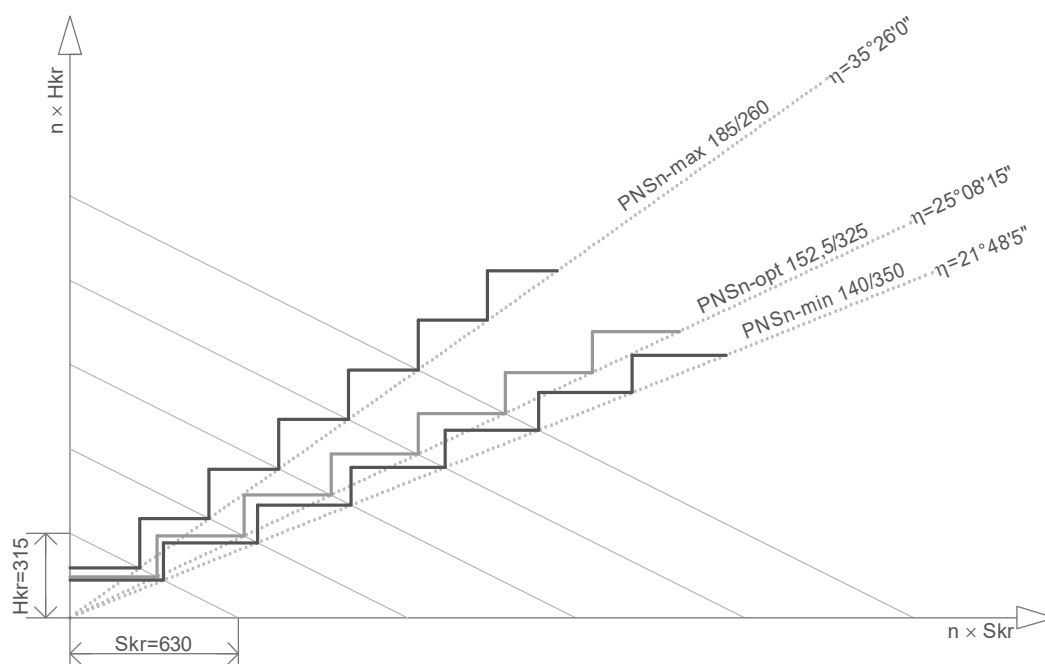
RYS. 3-4 PRZYKŁADOWE WYKRESY SCHODÓW NORMALNYCH
