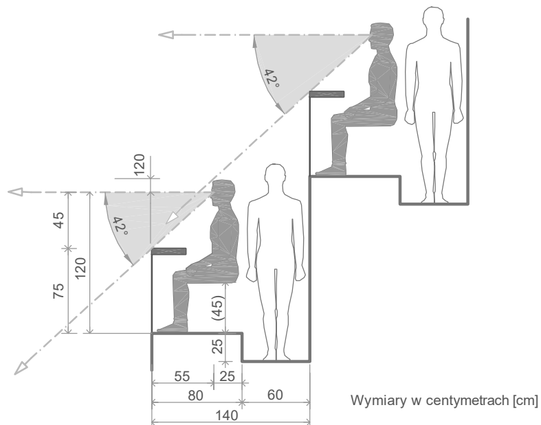
RYS. 5-2 TRYBUNA O PODWYŻSZONYM KOMFORTCIE UŻYTKOWYM - RZĄD Z BLATEM CZOŁOWYM I OBNIŻONYM PRZEJŚCIEM Z TYŁU
