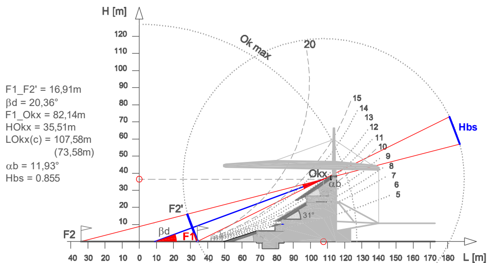
RYS. 2-17 STADE DE FRANCE - CHARAKTERYSTYKA PIONOWEGO PROFILU WIDOWNI
