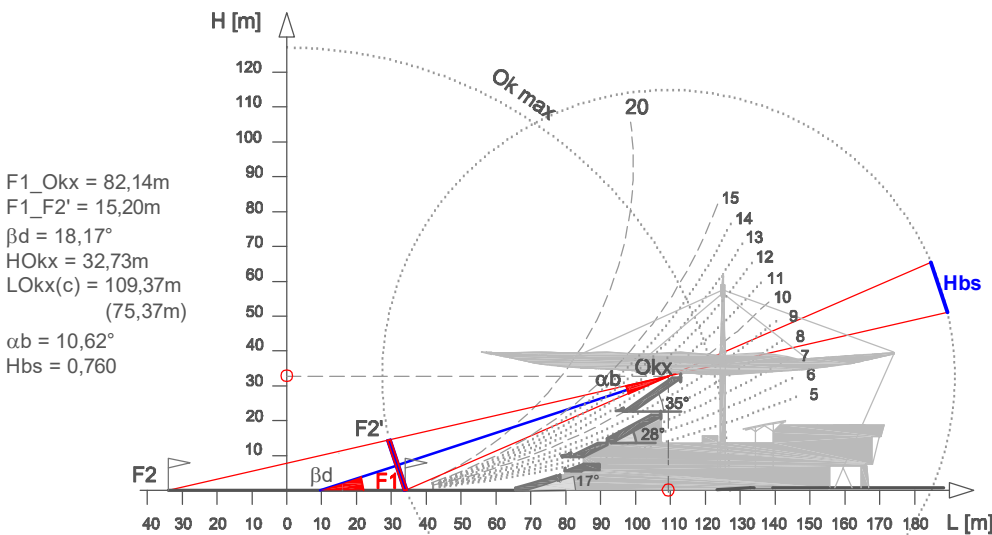
RYS. 2-18 STADION ŚLĄSKI - CHARAKTERYSTYKA PIONOWEGO PROFILU WIDOWNI (projektowana nadbudowa widowni wschodniej)
