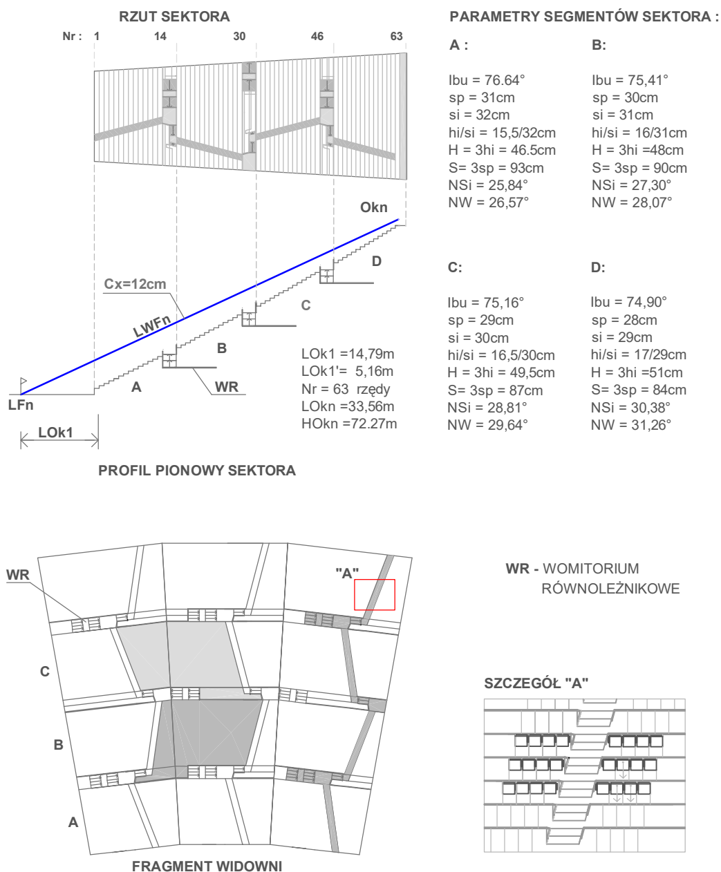
RYŚ. 5-14 PRZYKŁADOWA WIDOWNIA Z ZASTOSOWANIEM SCHODÓW UKOŚNYCH, NAPRZEMIENNEGO UKŁADU SIEDZISK I WOMITORIÓW RÓWNOLEŻNIKOWYCH.
