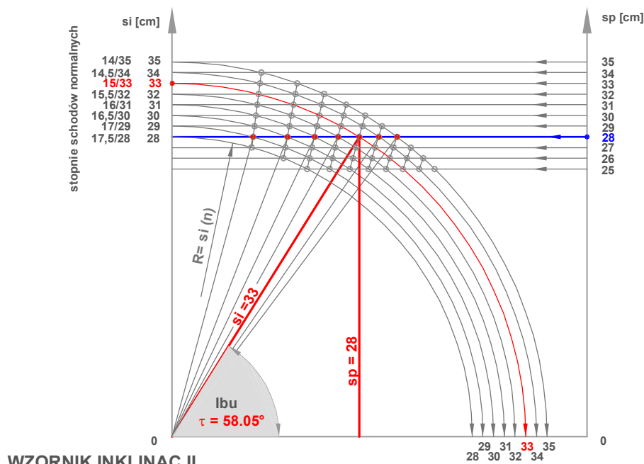
WZORNIK INKLINACJI
