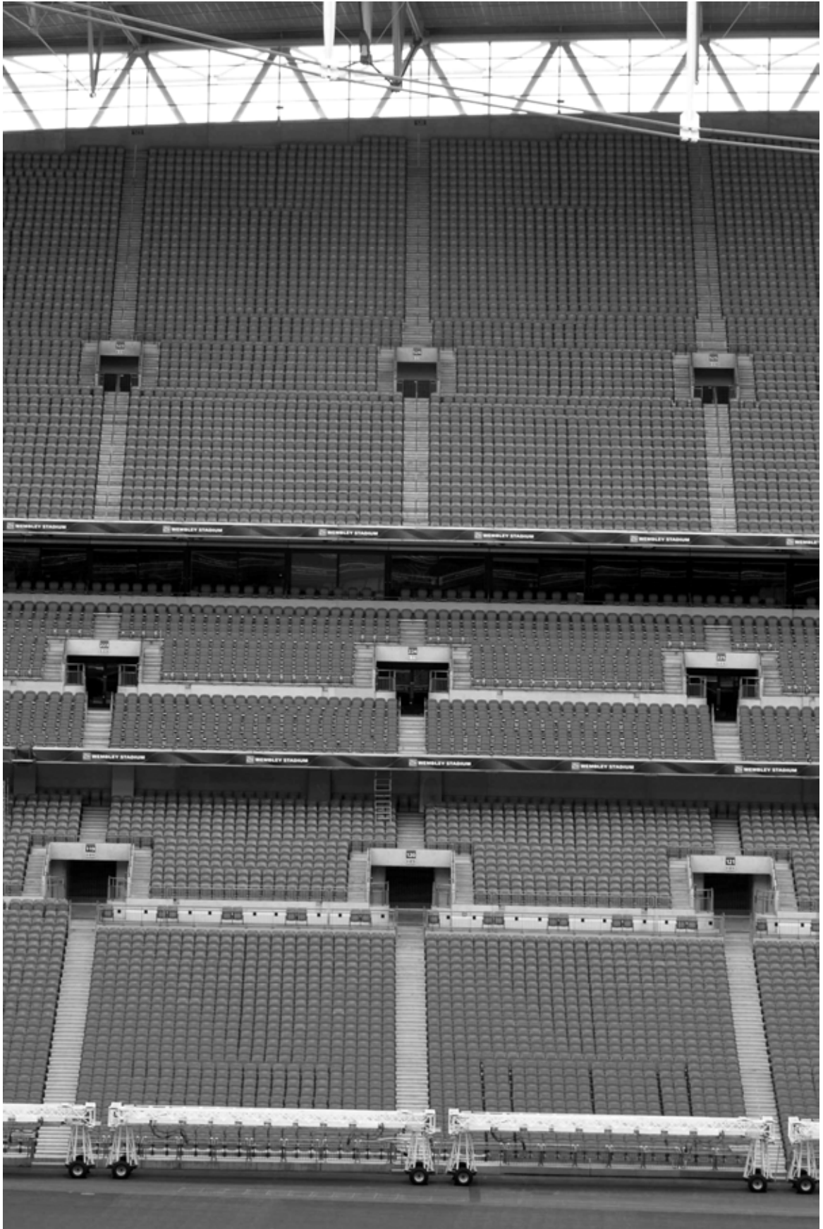
Fot. 4-1. Stadion Wembley (2008) – fragment widowni. Widoczny układ komunikacji i ewakuacji na poszczególnych piętrach trybun. Zróżnicowane szerokości wómitoriów decydują o różnych czasach ewakuacji osiąganych w obsługiwanych przez nie sektorach widowni.
